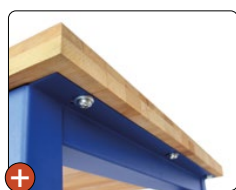
Les plateaux sont équipés d'inserts M8 afin de faciliter le montage
